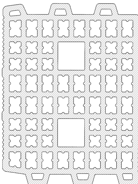
Caratteristiche geometriche dell'elemento
